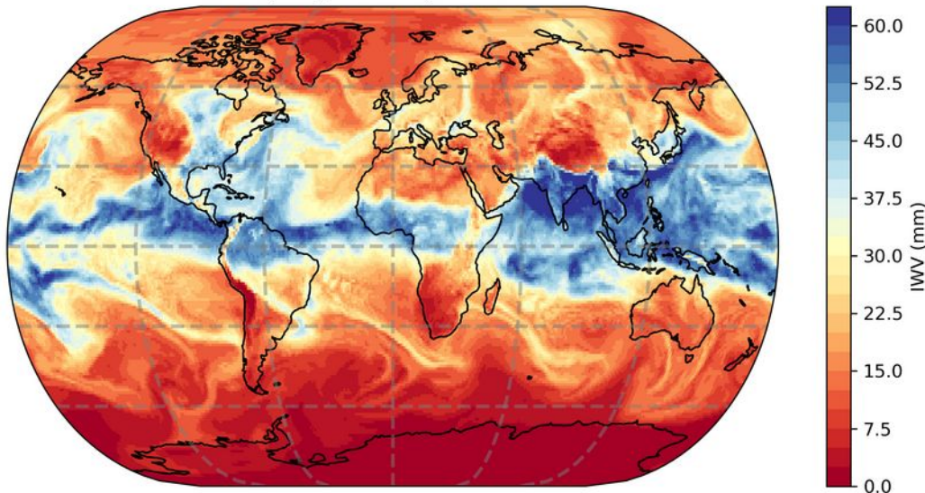
IWV (mm) summer, 01.07.2020
